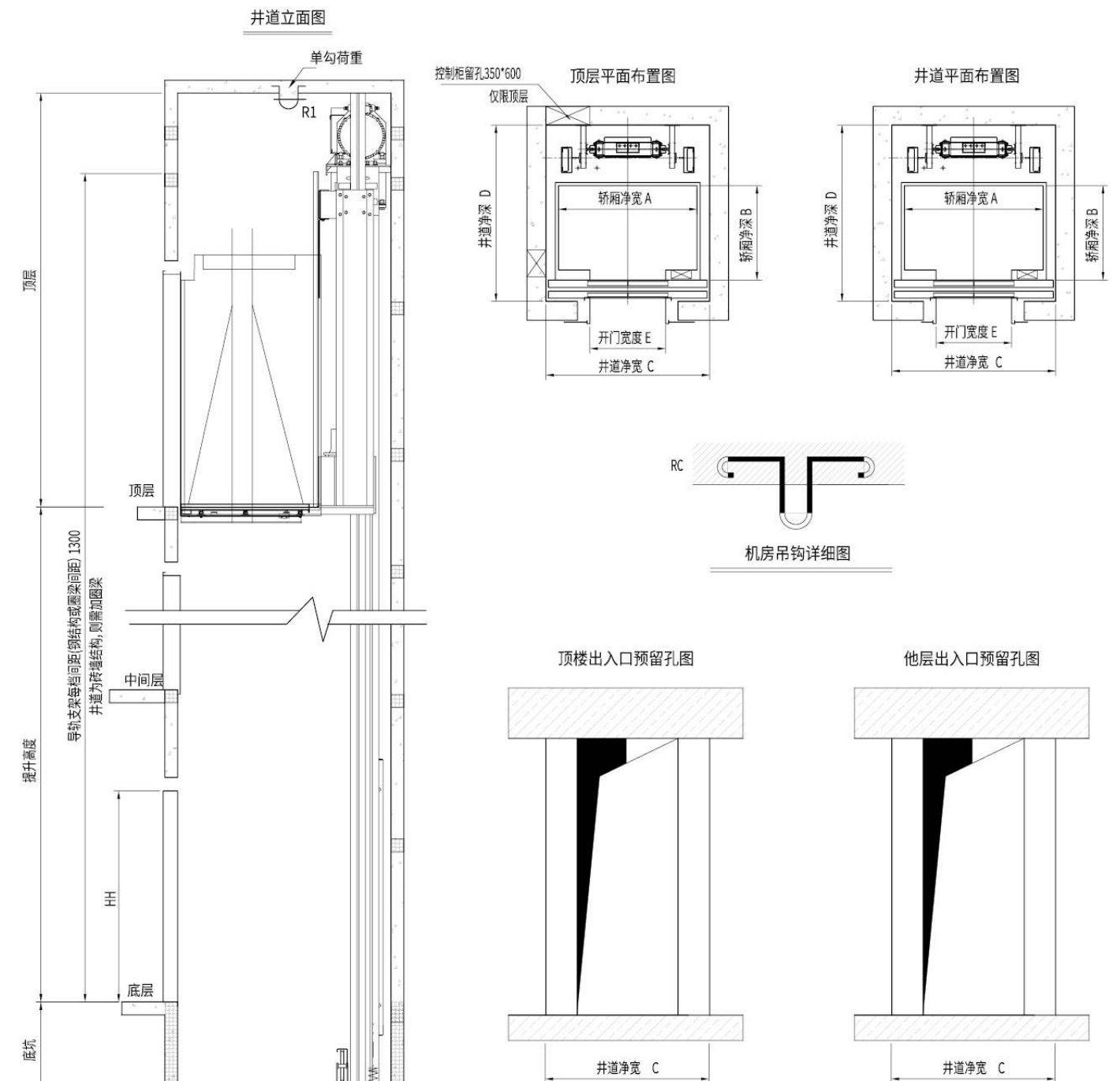
金泰系列土建示意图
