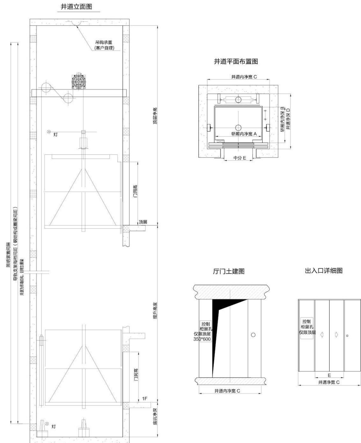
鸿泰系列土建示意图
