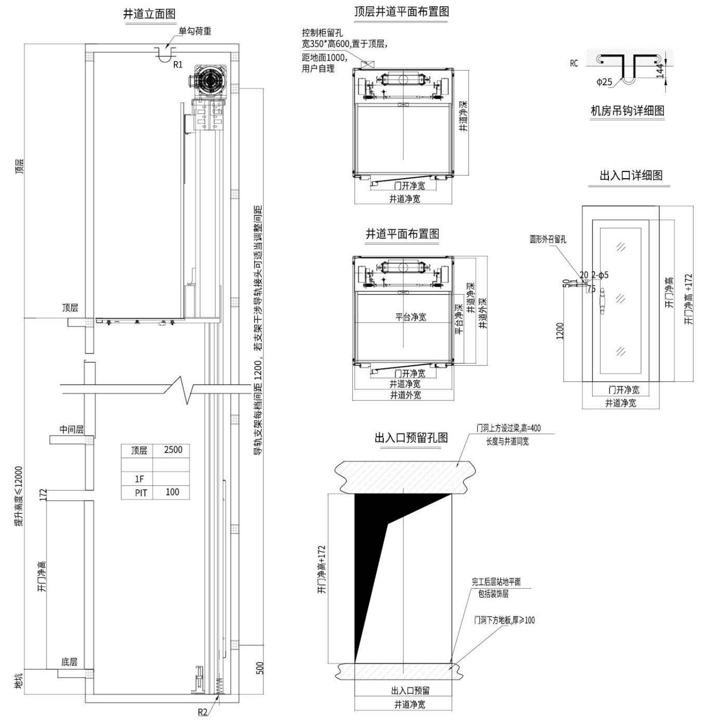
泰山+系列土建示意图
