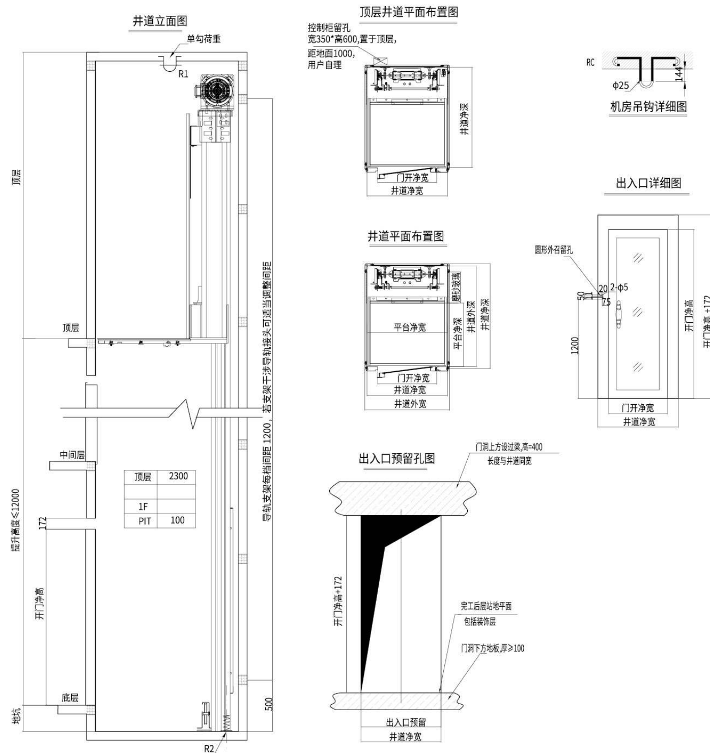
泰山 A 系列土建示意图
